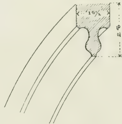
Fig. 7. Przekrój żebra.
